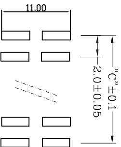
P.C.B LAYOUT
